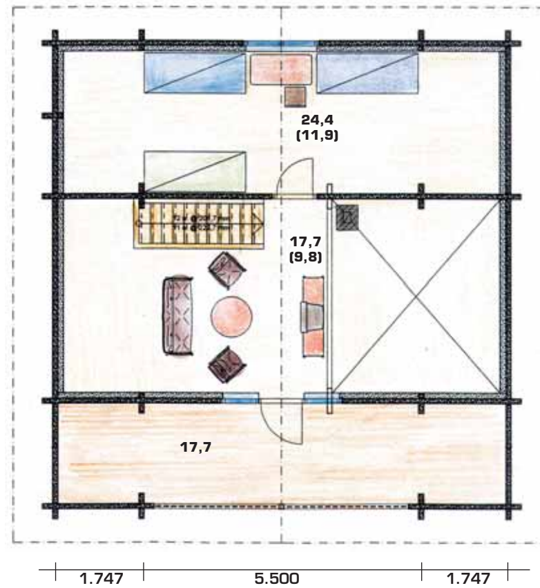
Parvi • Loft
