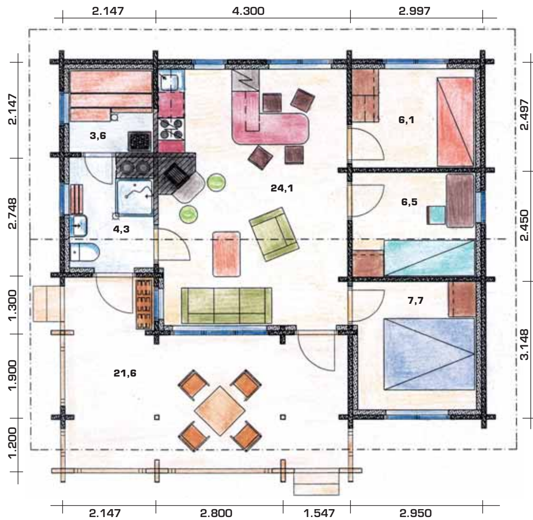
Alakerta • Bottenvåning
