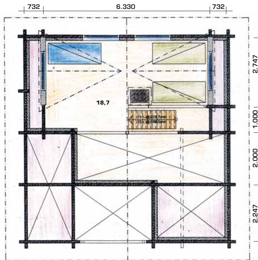
Parvi • Loft
