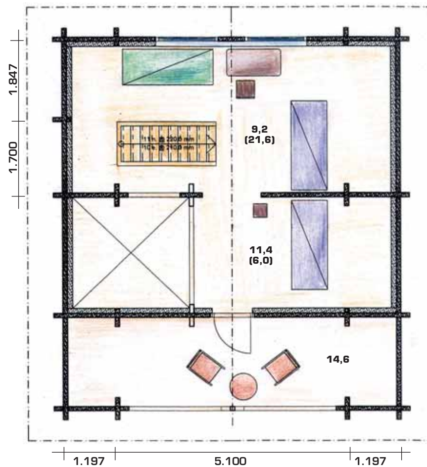
Parvi • Loft
