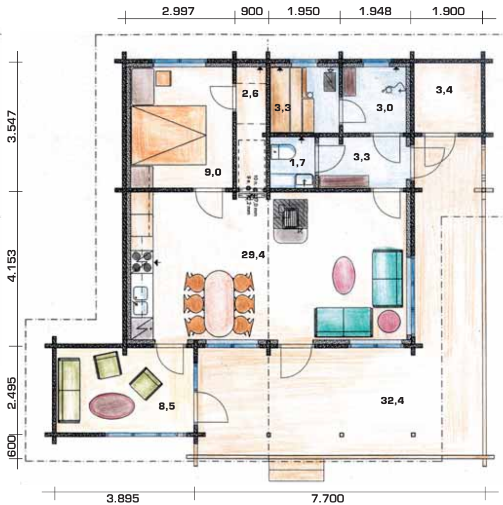
Alakerta • Bottenvåning
