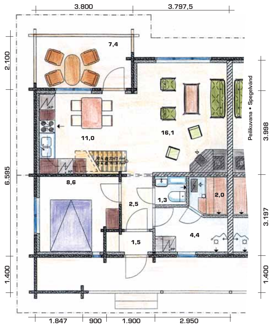
Alakerta • Bottenvåning
