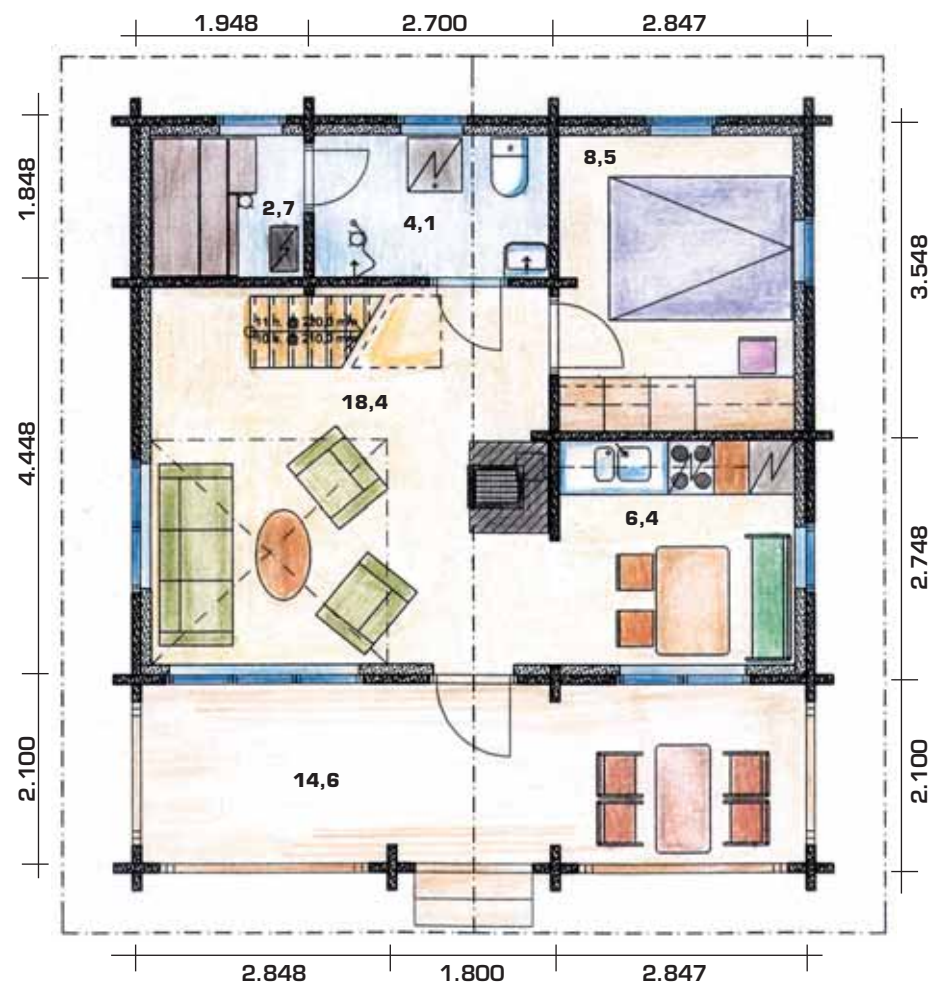
Alakerta • Bottenvåning
