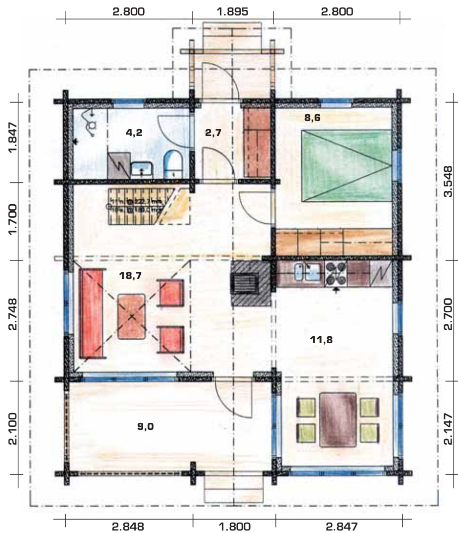
Alakerta • Bottenvåning
