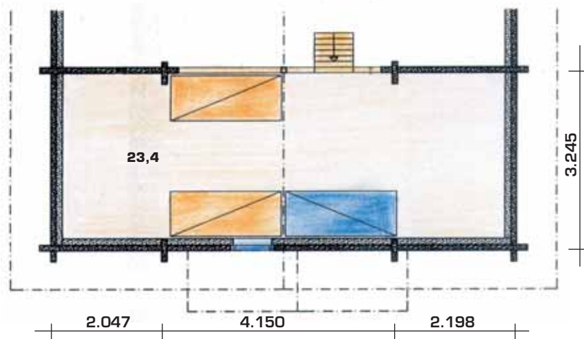
Parvi • Loft
