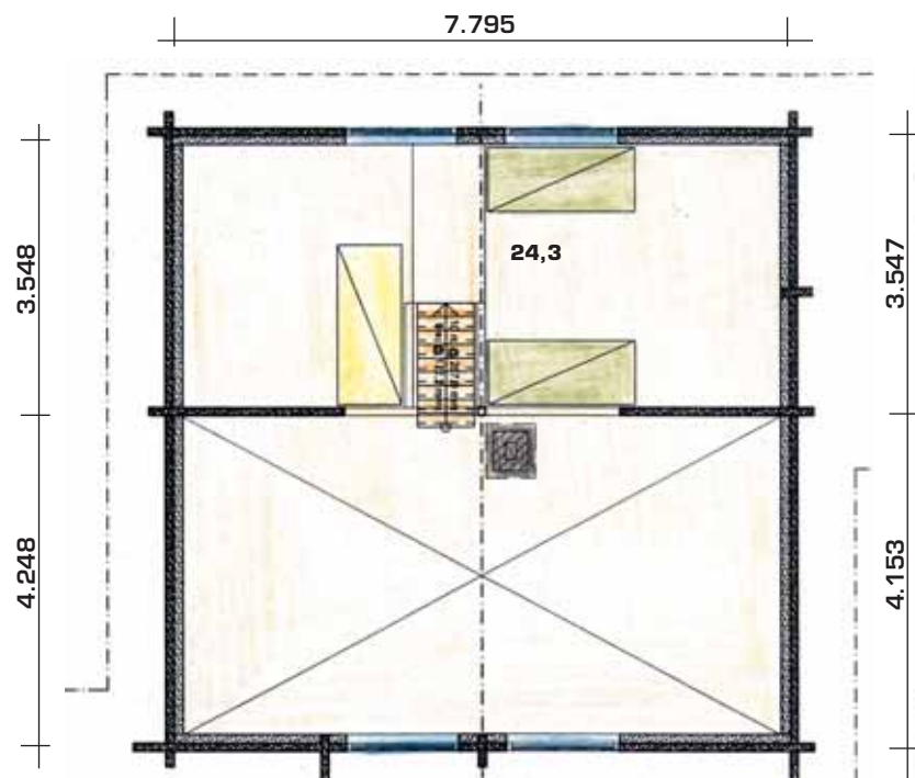
Parvi • Loft
