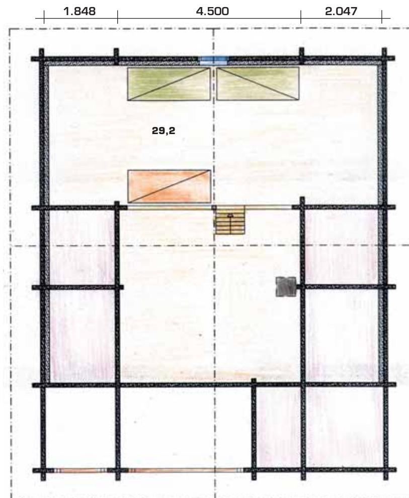
Parvi • Loft
