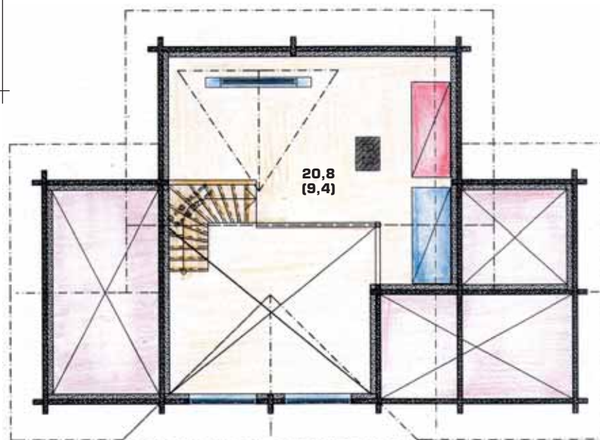
Parvi • Loft
