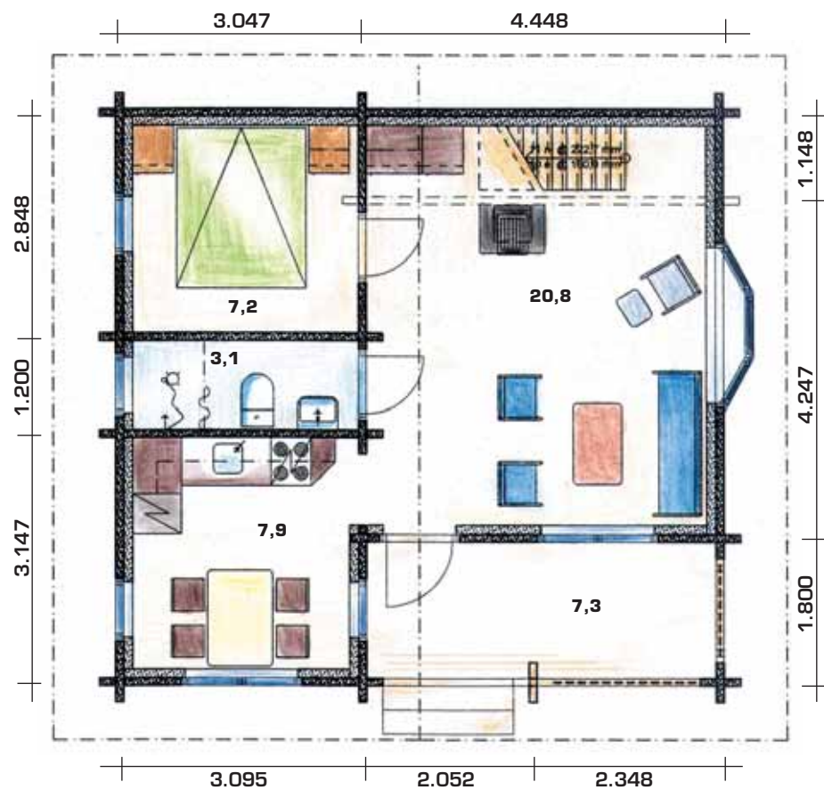
Alakerta • Bottenvåning
