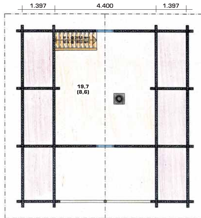
Parvi • Loft
