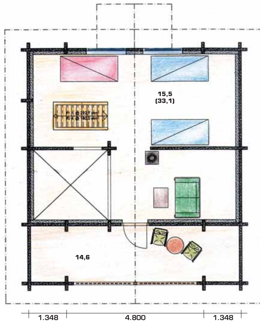
Parvi • Loft
