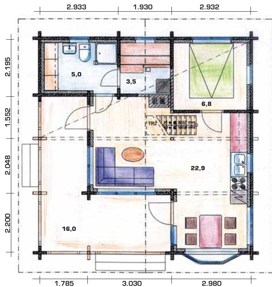
Alakerta • Bottenvåning
