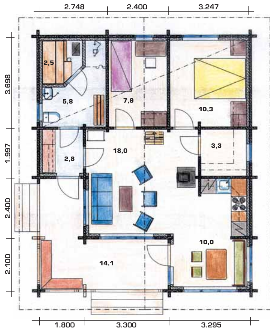
Alakerta • Bottenvåning
