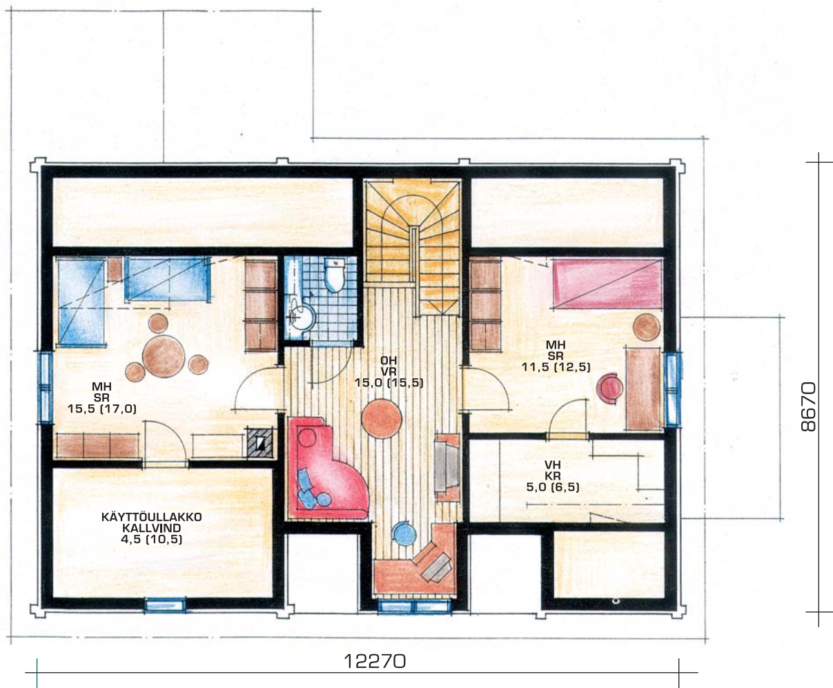
Yläkerta • Övre våning
